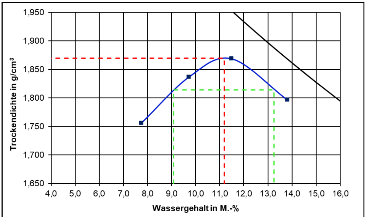
Proctorkurve des untersuchten RC-Materials 0/45 mm (aus Prüfbericht F 21/01/0114 – IV/2020)
